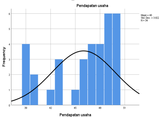
Gambar 2. Histogram Variabel Pendapatan Usaha (Y)
