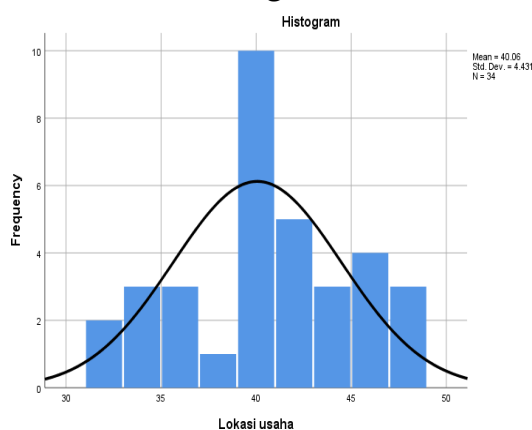
Gambar 1. Histogram Lokasi Usaha (X)
