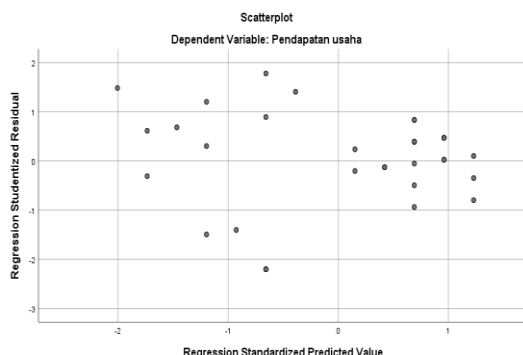
Gambar 4. Uji Heteroskedastisitas
