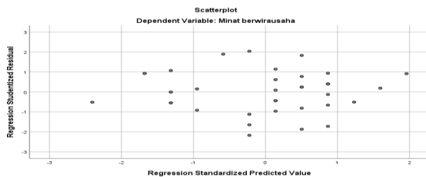
Gambar 4 Uji Heteroskedastisitas
