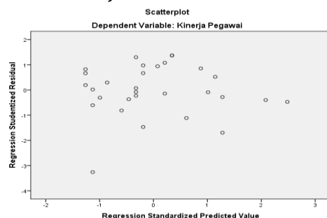
Gambar 1. Uji Heteroskedastisitas
